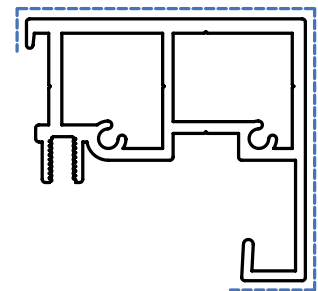
Guide rail (7-303770-0000)
