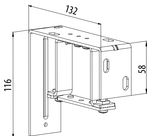
Fixed hanger (vnitřní věšák Al) 132 mm P011 (2-00384) (for head rail 58 x 60)
