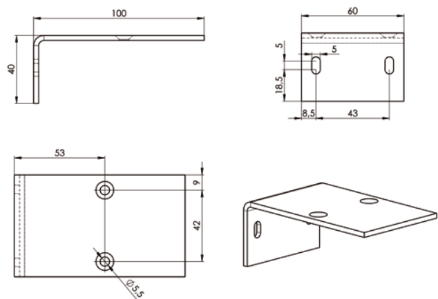
Guide rail (7-303770-0000)
