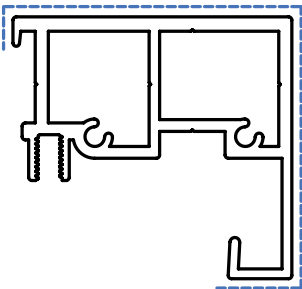
Guide rail (7-303770-0000)
