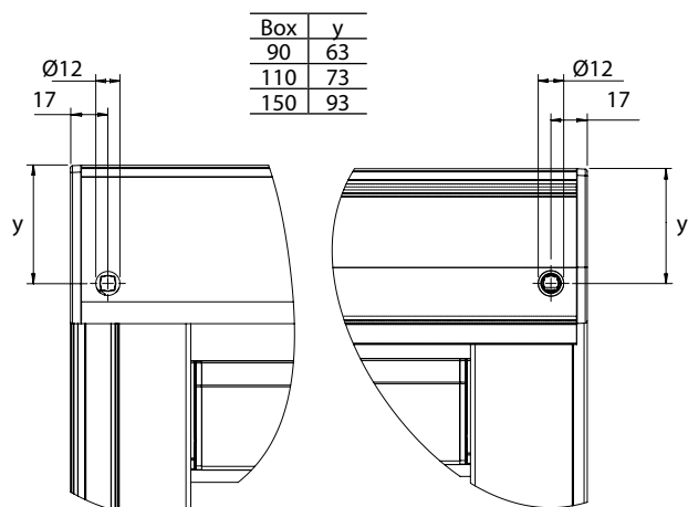
detachable crank 90° outlet O
