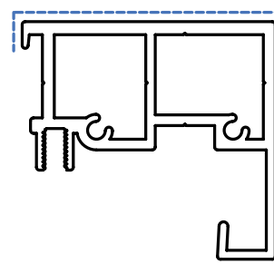
Guide rail (7-303770-0000)
